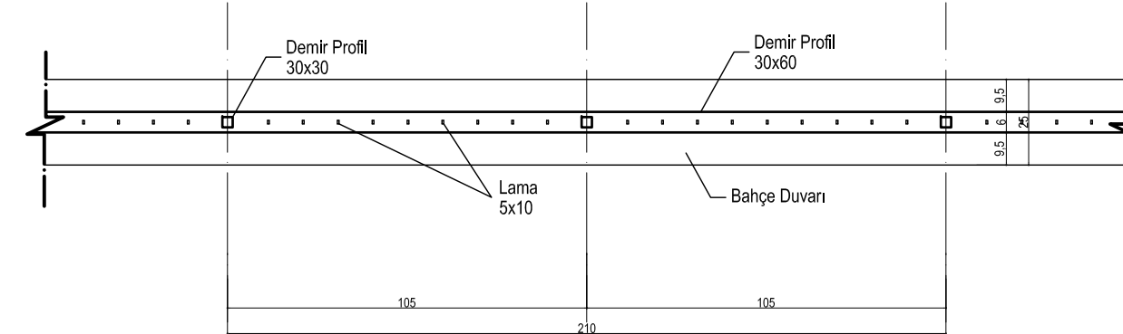
BAHÇE DUVARI PLAN Ölçek: 1/20
