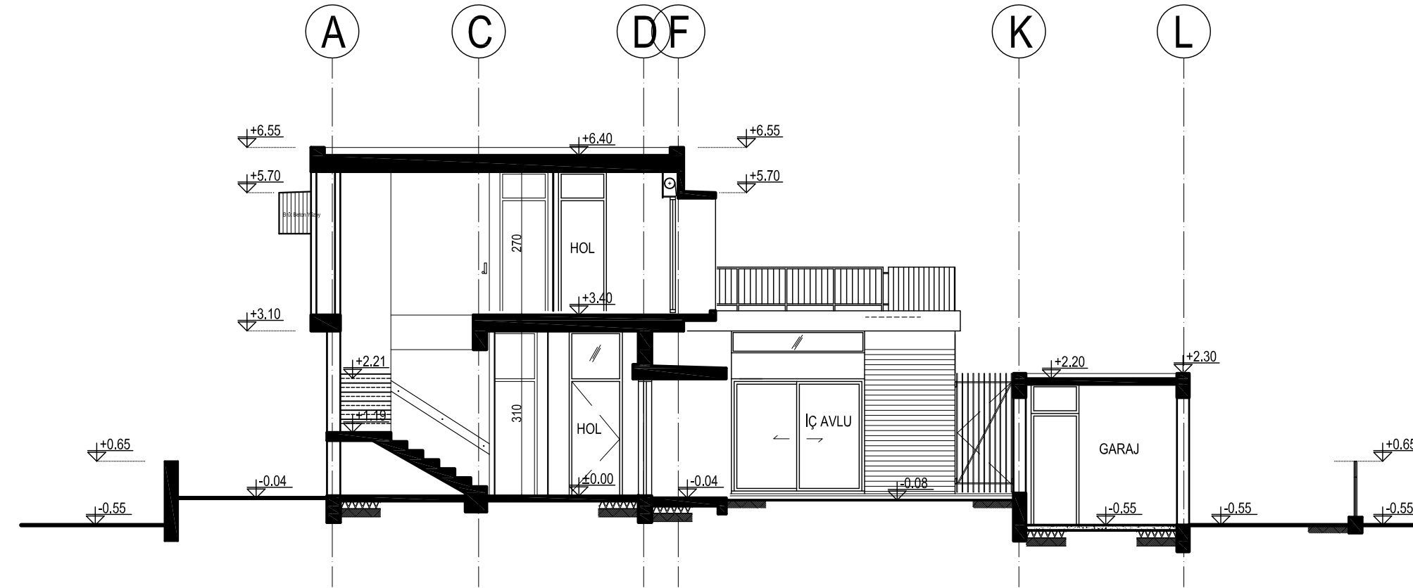
A-A KESİTİ Ölçek: 1/100
