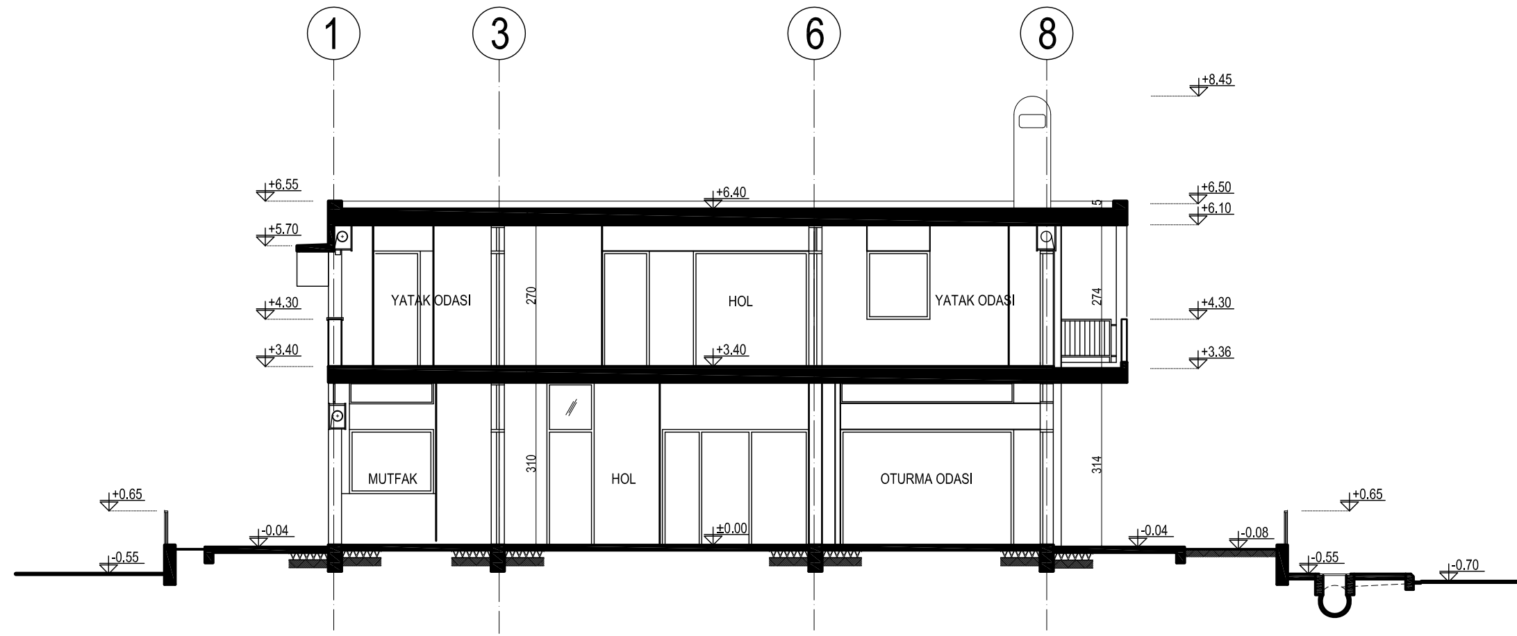
B-B KESİTİ Ölçek: 1/100
