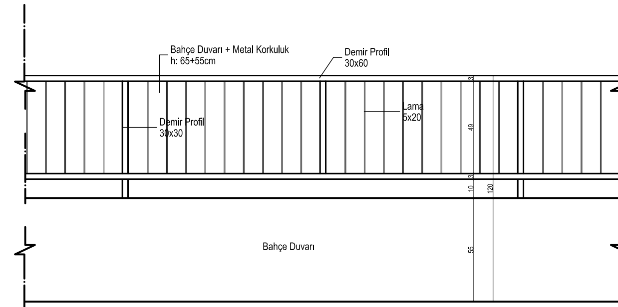
BAHÇE DUVARI ÖN GÖRÜNÜŞ Ölçek: 1/20
