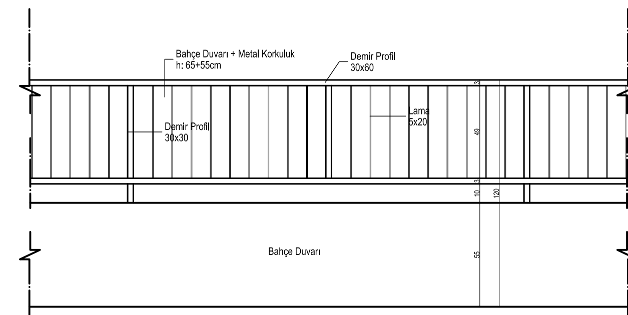
BAHÇE DUVARI ÖN GÖRÜNÜŞÜ Ölçek: 1/20
