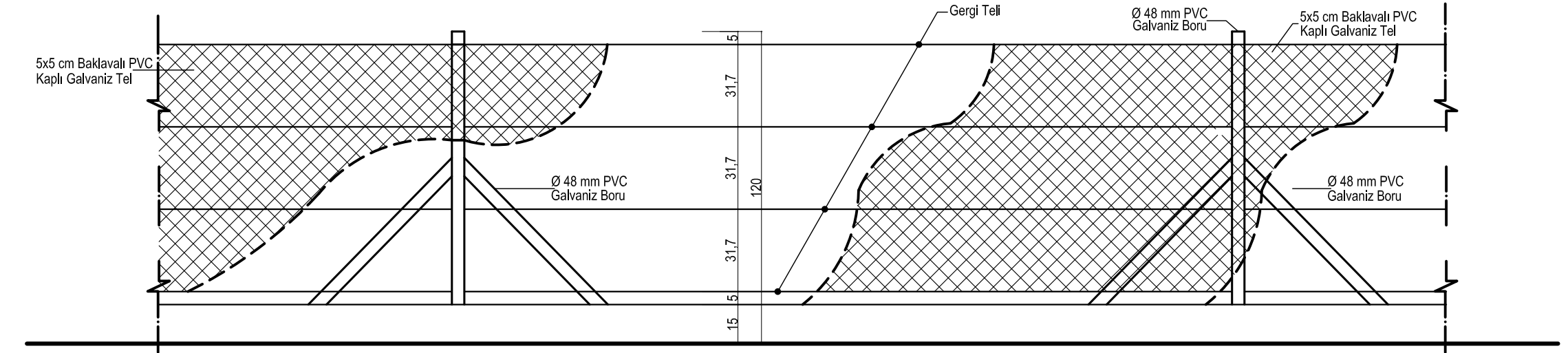
TELLEME ÖN GÖRÜNÜŞÜ Ölçek: 1/20
