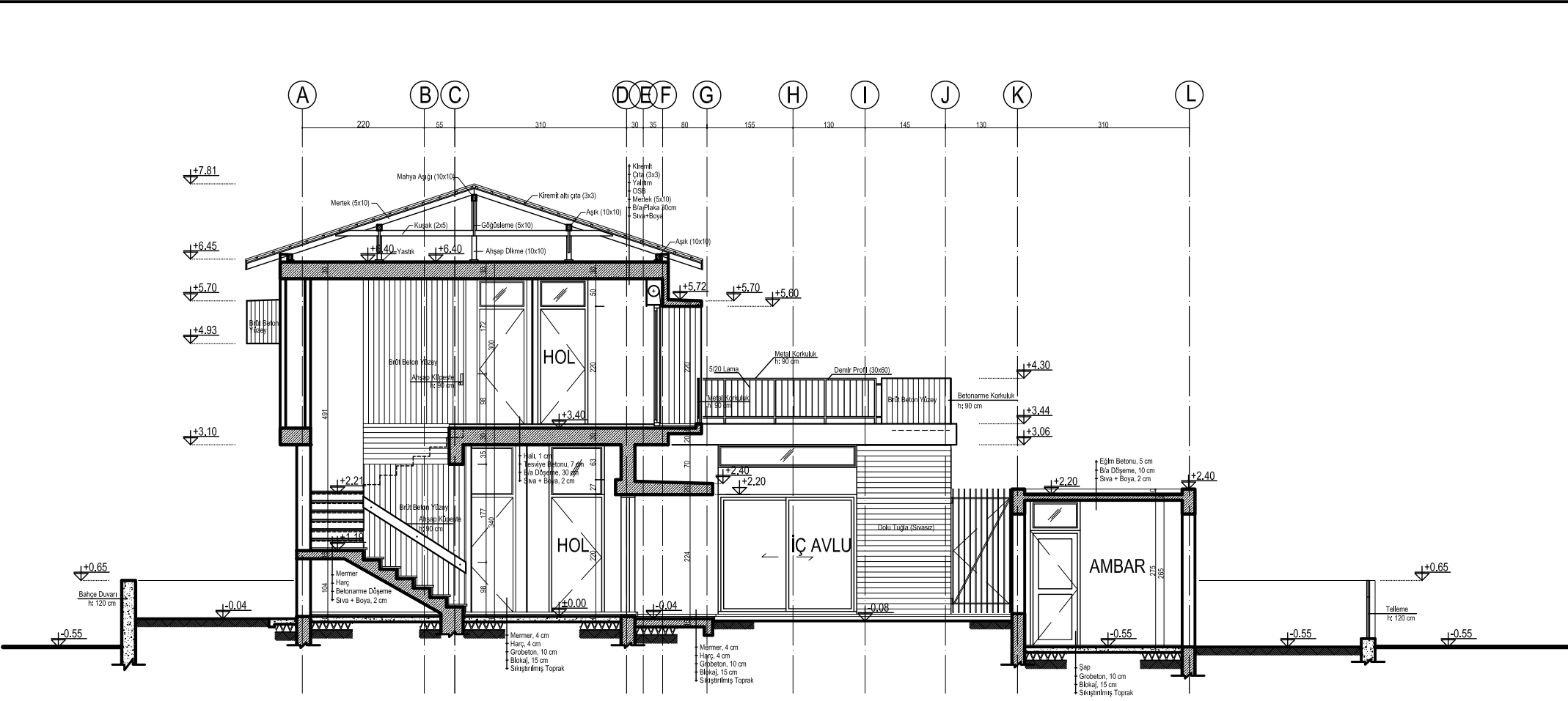
A-A KESİTİ Ölçek: 1/100
