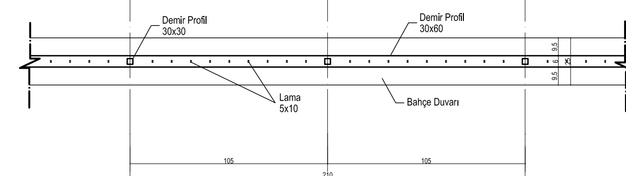
BAHÇE DUVARI PLAN Ölçek: 1/20
