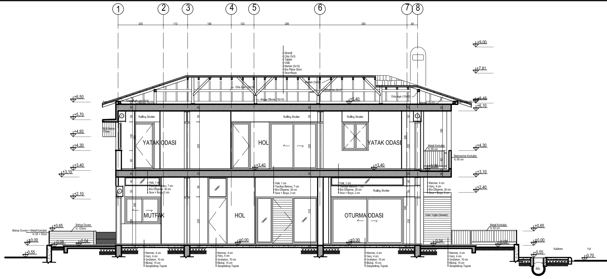
B-B KESİTİ Ölçek: 1/100
