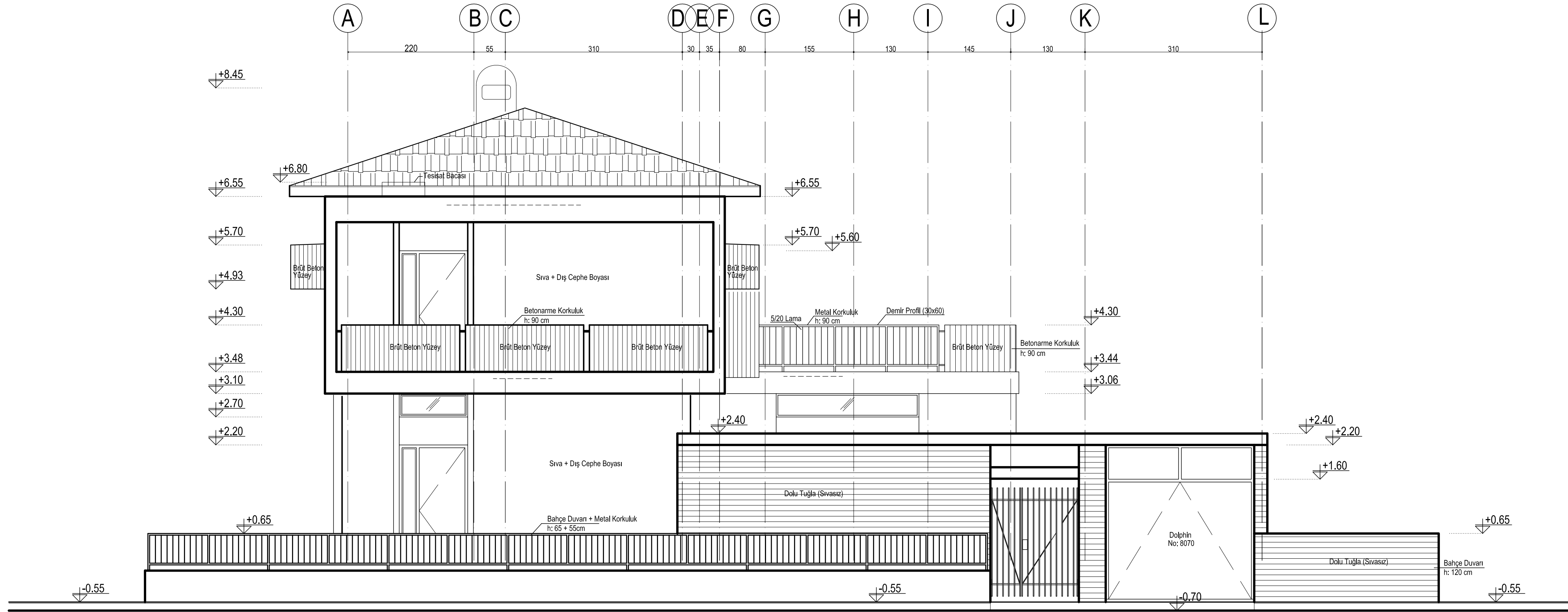
KUZEY CEPHESİ ÖLÇEK:1/50
