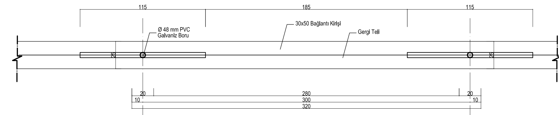
TELLEME PLAN Ölçek: 1/20
