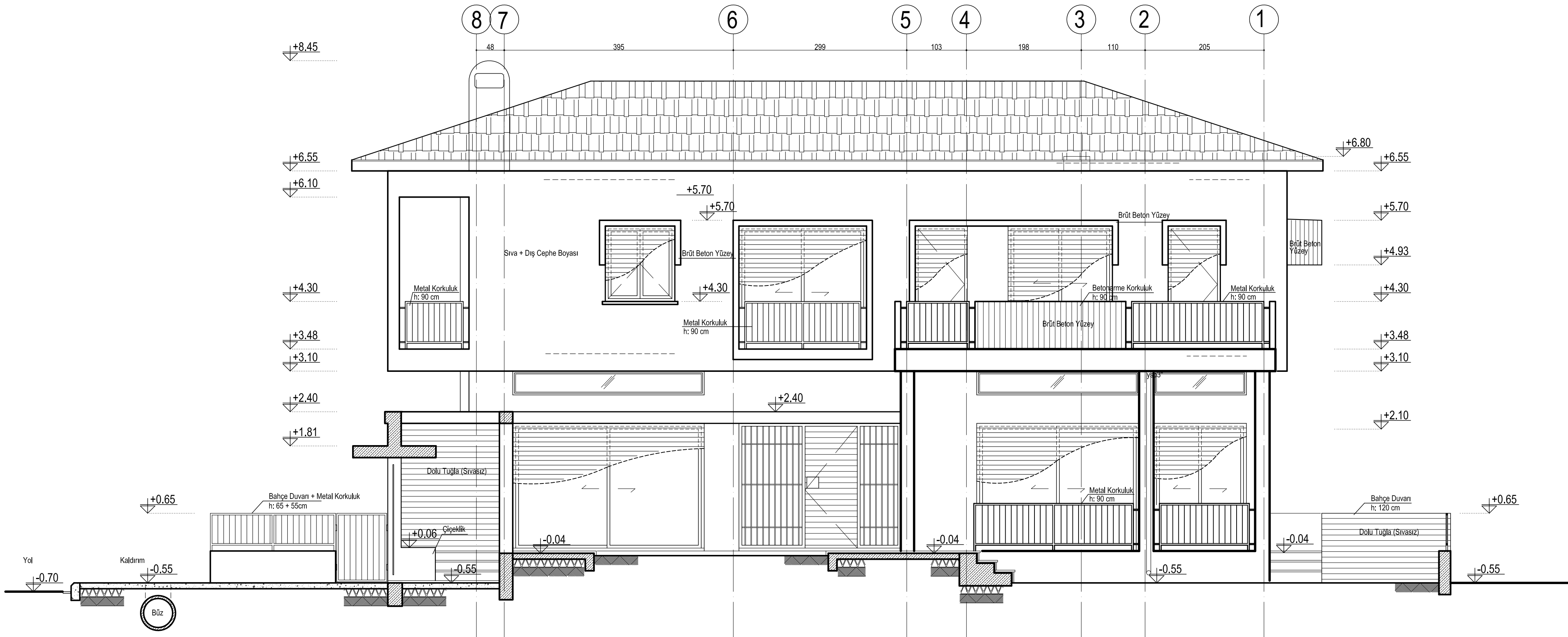
BATI CEPHESİ ÖLÇEK:1/50
